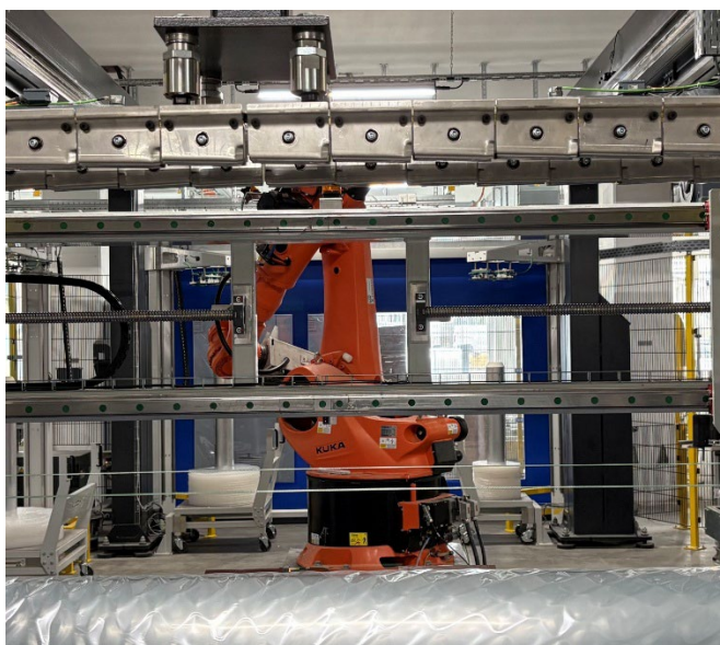
Modernste automatisierte Packerei der neuen HOSTAPHAN™ Polyesterfolien-Anlage
